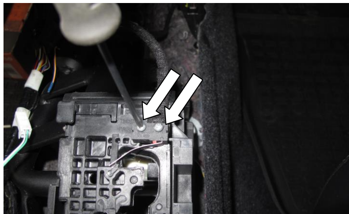
Установите концевик жгута проводов (поз. 10) на селекторе закрепив винтами (поз. 6)
